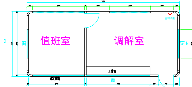
平面布局图
